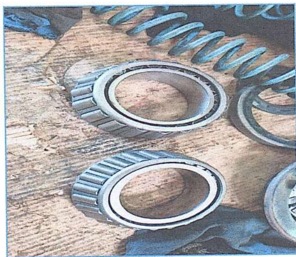
IMAGENS DETALHADAS DE COMPONENTES INTERNOS DO CONJUNTO DIFERENCIAL ONDE PODEMOS VER CLARAMENTE DESGASTE E AVARIAS ESTRUTURAIS
