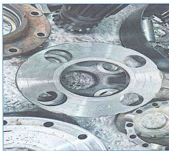
IMAGENS DETALHADAS DE COMPONENTES INTERNOS DO CONJUNTO DIFERENCIAL ONDE PODEMOS VER CLARAMENTE DESGASTE E AVARIAS ESTRUTURAIS
