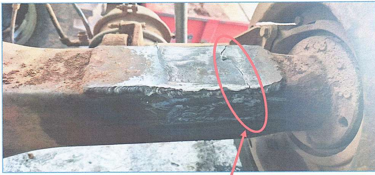
IMAGEM DETALHADA DE TRINCA JUNTO AO DIFERENCIAL, MUITAS SOLDAS JÁ EXECUTADAS NO MESMO
