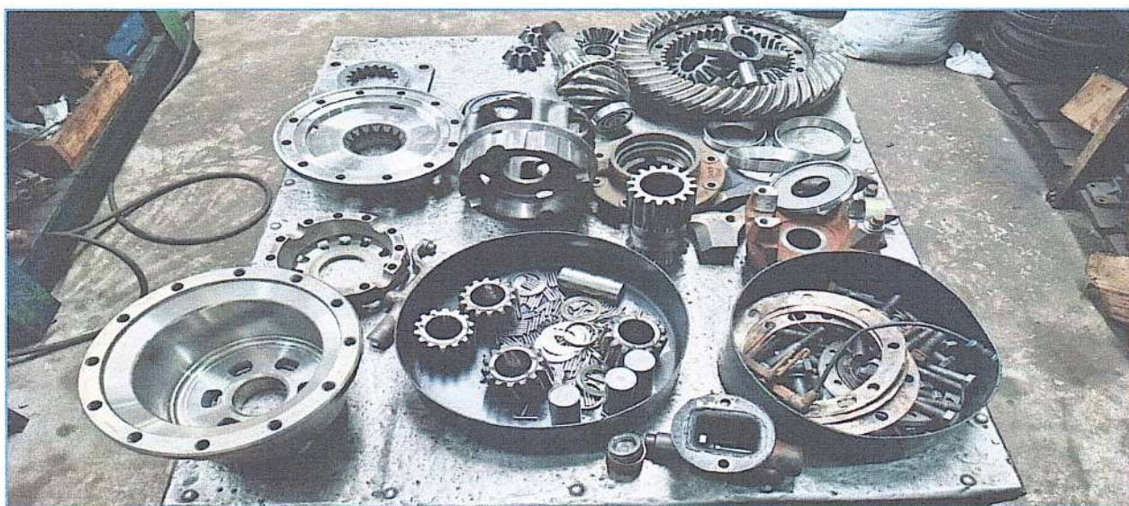
IMAGEM DOS INTERNOS DO CONJUNTO DE DIFERENCIAL DESMONTADOS PARA INSPEÇÃO
