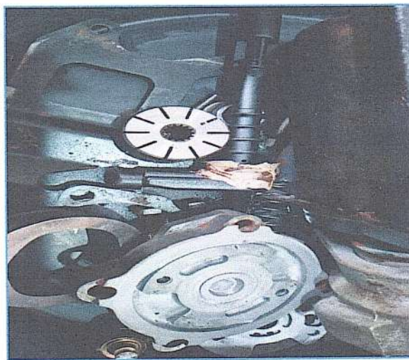
IMAGEM DA BOMBA DA DIREÇÃO HIDRÁULICA JÁ DESMONTADA PARA INSPEÇÃO
