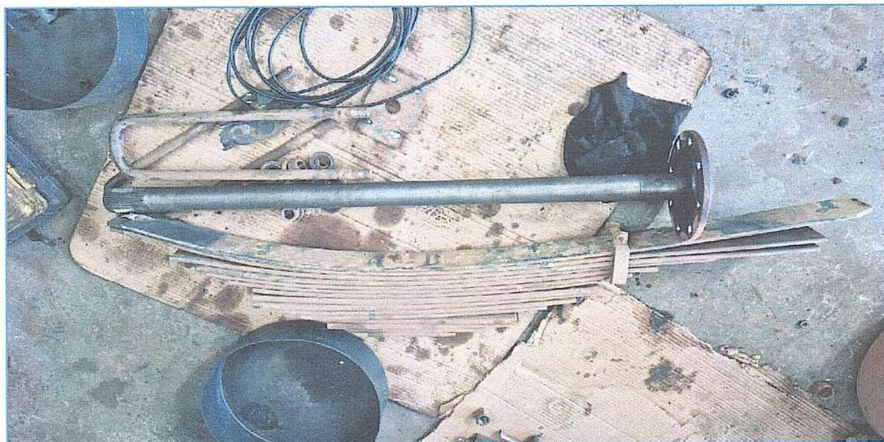
COMPONENTES DO EIXO TRASEIRO E FEIXE DE MOLAS DO VEÍCULO IVECO EUROCARGO REMOVIDOS PARA ANÁLISE DE DESGASTE E CONFERÊNCIA DE MEDIDAS.
